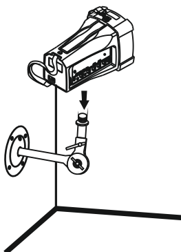
Bild 39: Wandhalterung MS-90
